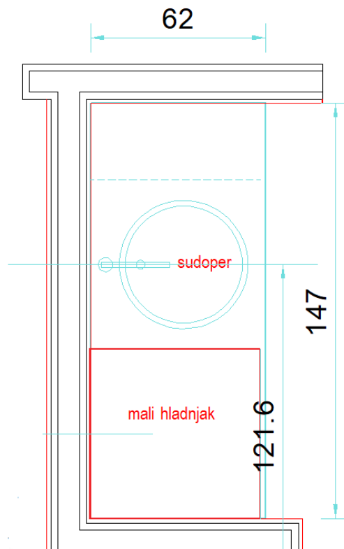
Grupa 10.1. – Pozicija 28. – Skica 2
