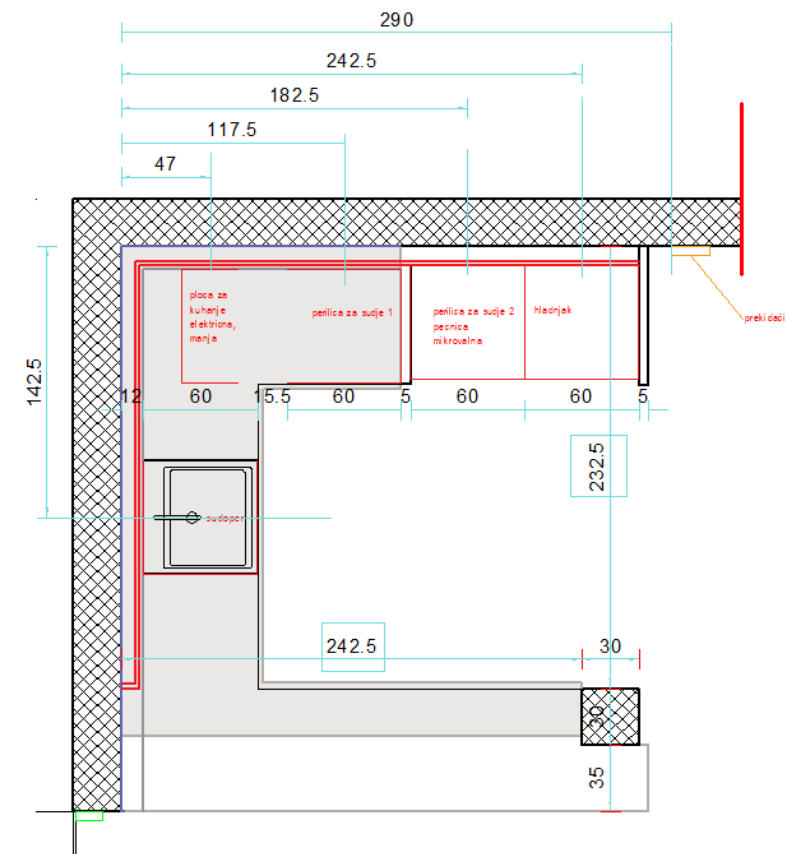
Grupa 10.1. – Pozicija 31. – Skica 4
